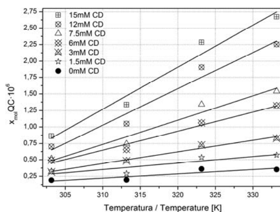
Rys. 2. Rozpuszczalność QC w roztworach CD
